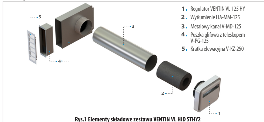
Rys.1 Elementy składowe zestawu VENTIN VL HID STHY2
