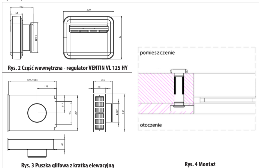
Rys. 3 Puszka glifowa z kratką elewacyjną
