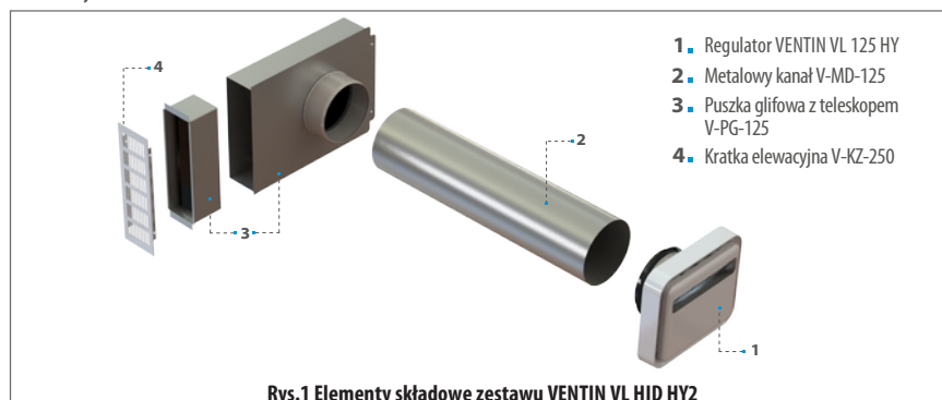
Rys.1 Elementy składowe zestawu VENTIN VL HID HY2
