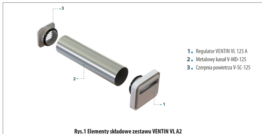
Rys.1 Elementy składowe zestawu VENTIN VL A2
