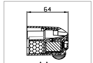
RYS. 2 Przekrój
