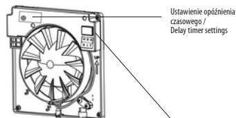
Rys 5. / Pict 5. - Dostęp do połączeń elektrycznych / Access to electrical connections
