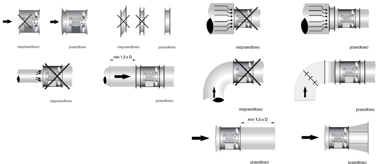
PRZYKŁAD MONTAŻU WENTYLATORÓW OSIOWYCH
