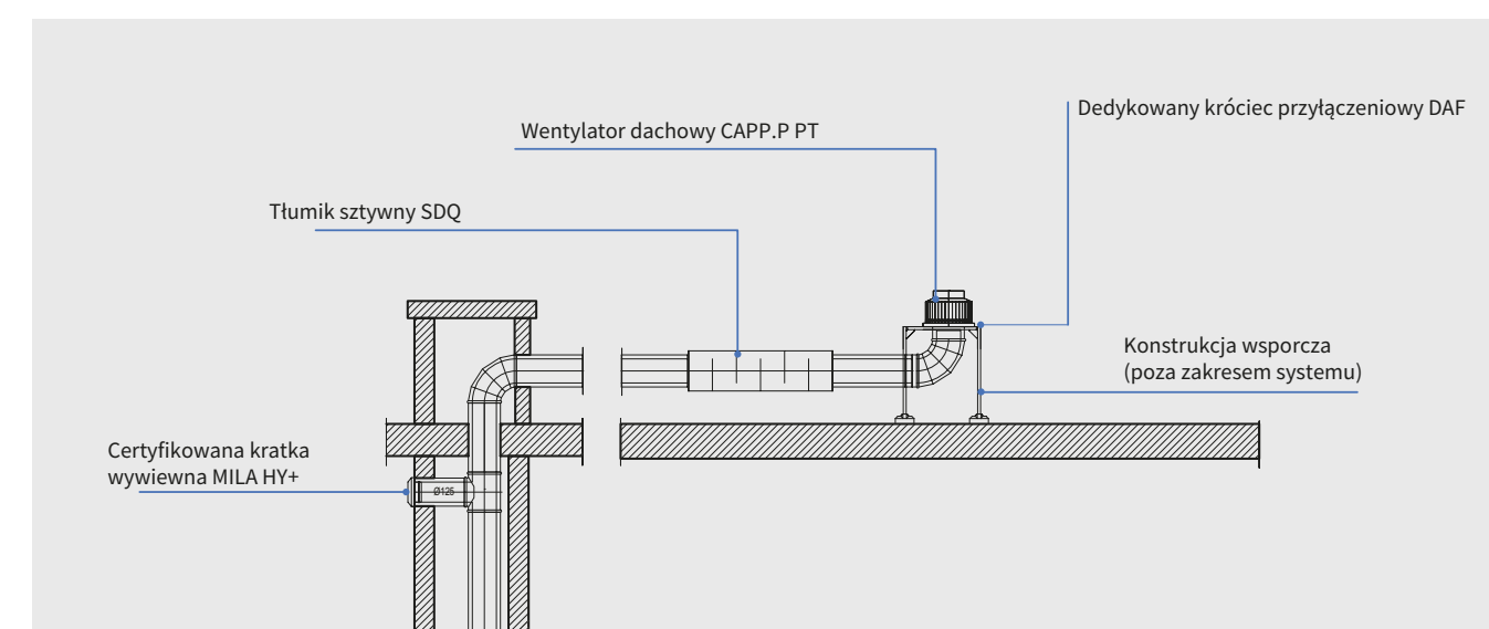
Przykład montażu wentylatora bez podstawy dachowej z dedykowanym króćcem przyłączeniowym oraz sztywnym tłumikiem
