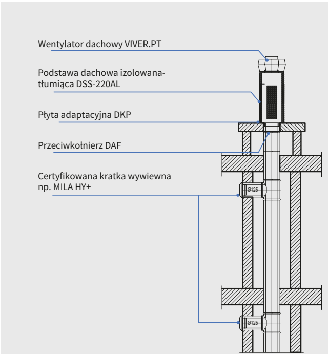
Wentylator dachowy z podstawą tłumiącą
