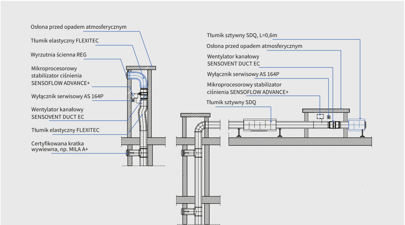
Przy podwyższonych wymaganiach akustycznych np. lokalizacja w bliskiej odległości okien lub tarasów, tłumiki stosowane mogą być również po stronie wylotu wentylatora
