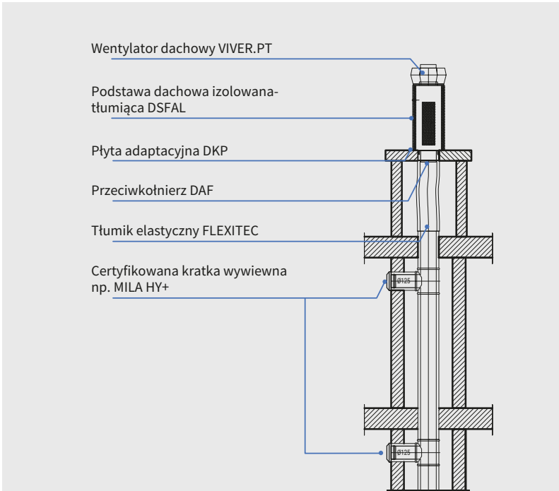
Wentylator dachowy z podstawą tłumiącą i tłumikiem elastycznym
