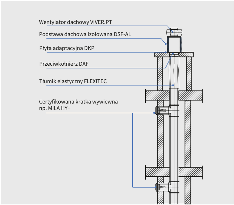
Wentylator dachowy z podstawą standardową- izolowaną oraz tłumikiem elastycznym
