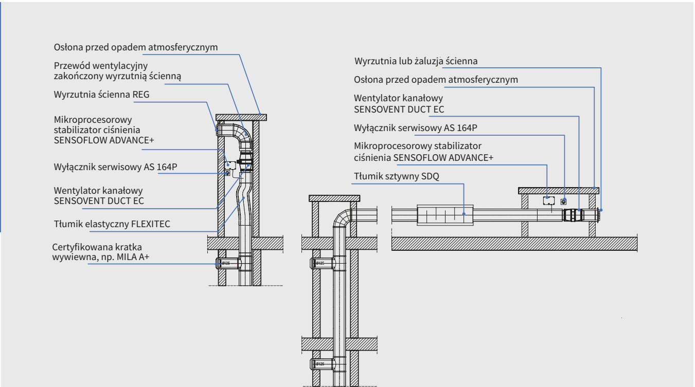
Wentylatory kanałowe w systemie sensovent® projektowane są zawsze wraz z tłumikami akustycznymi montowanymi po stronie ssawnej urządzenia
